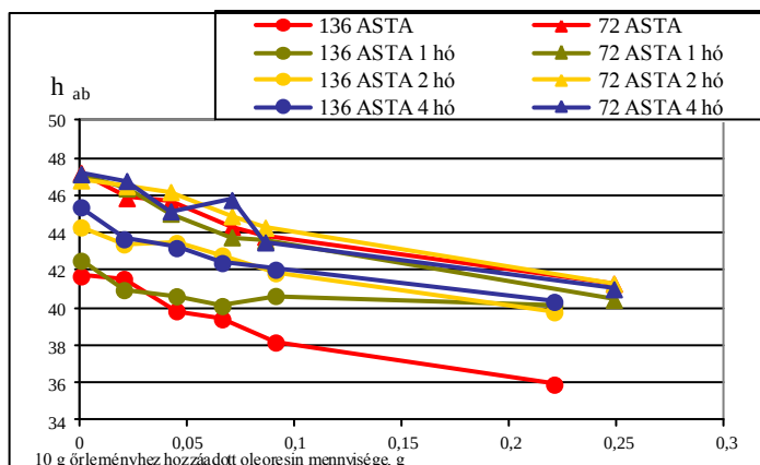
7. ábra A h_{ab}^o színezeti szög értékének alakulása a színezéktartalom növelése hatására
