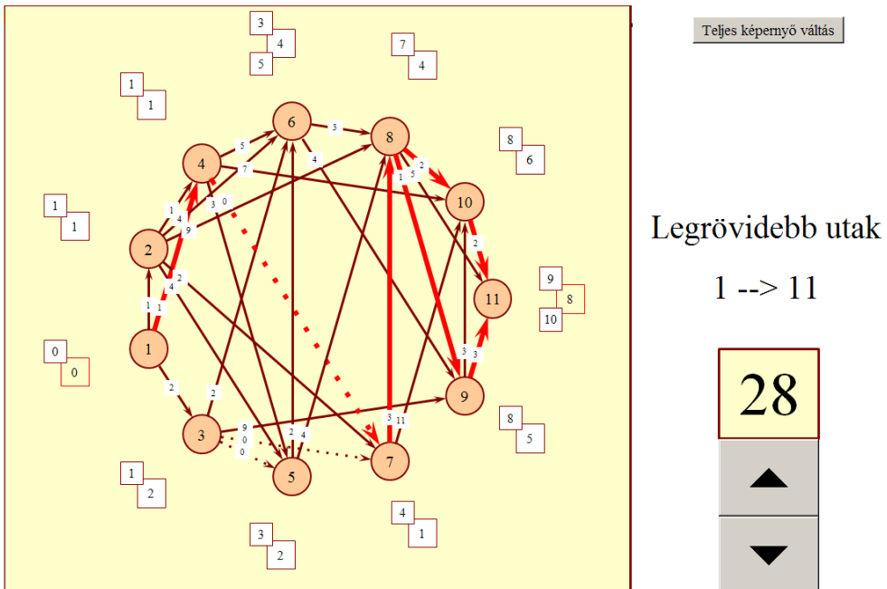
4. ábra: Legrövidebb utak keresése léptetéssel, végső állapot.
